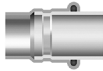
Przekrój połączenia po zaprasowaniu
