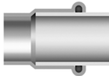
Przekrój połączenia przed zaprasowaniem
