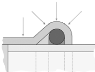
rys. Kierunki nacisku w połączeniu „press”
